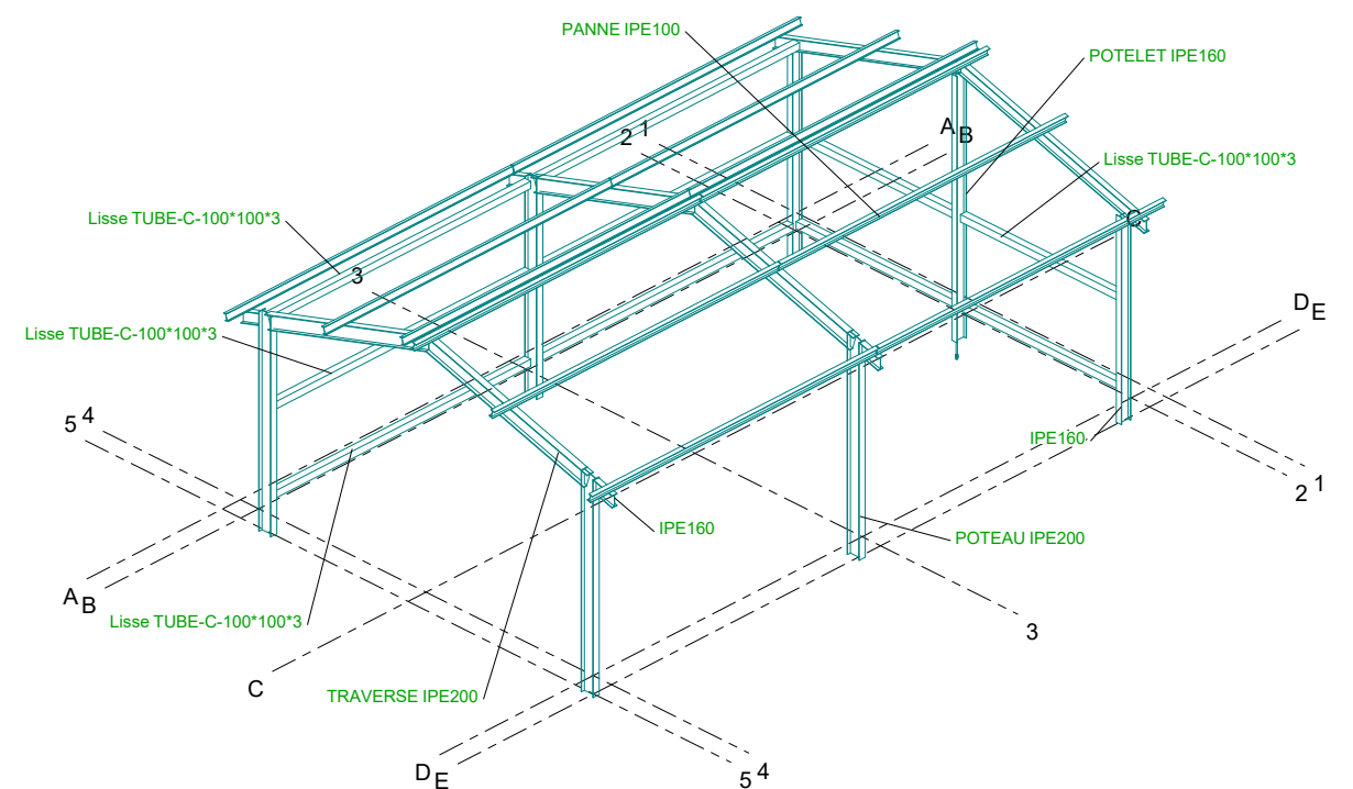
Toiture 1:100
