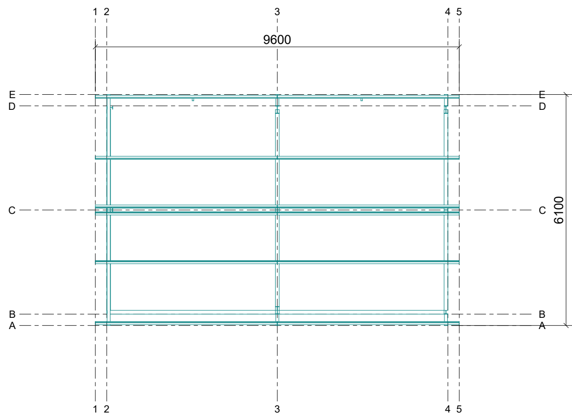
Toiture 1:100
