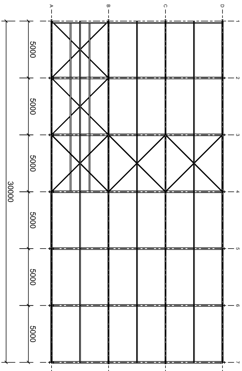
Plan 0.00 1:200
